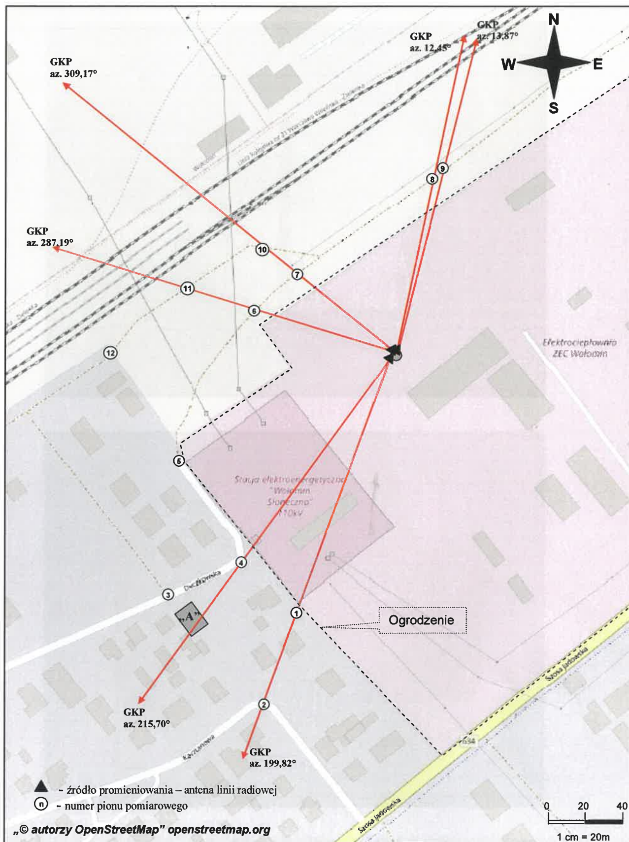
Rys. 1. Usytuowanie punktów i pionów pomiarowych w otoczeniu instalacji radiokomunikacyjnej Stacja Netia WOLOW001-WOLOM00001 Nowe Lipiny, ul. Szosa Jadowska 49
